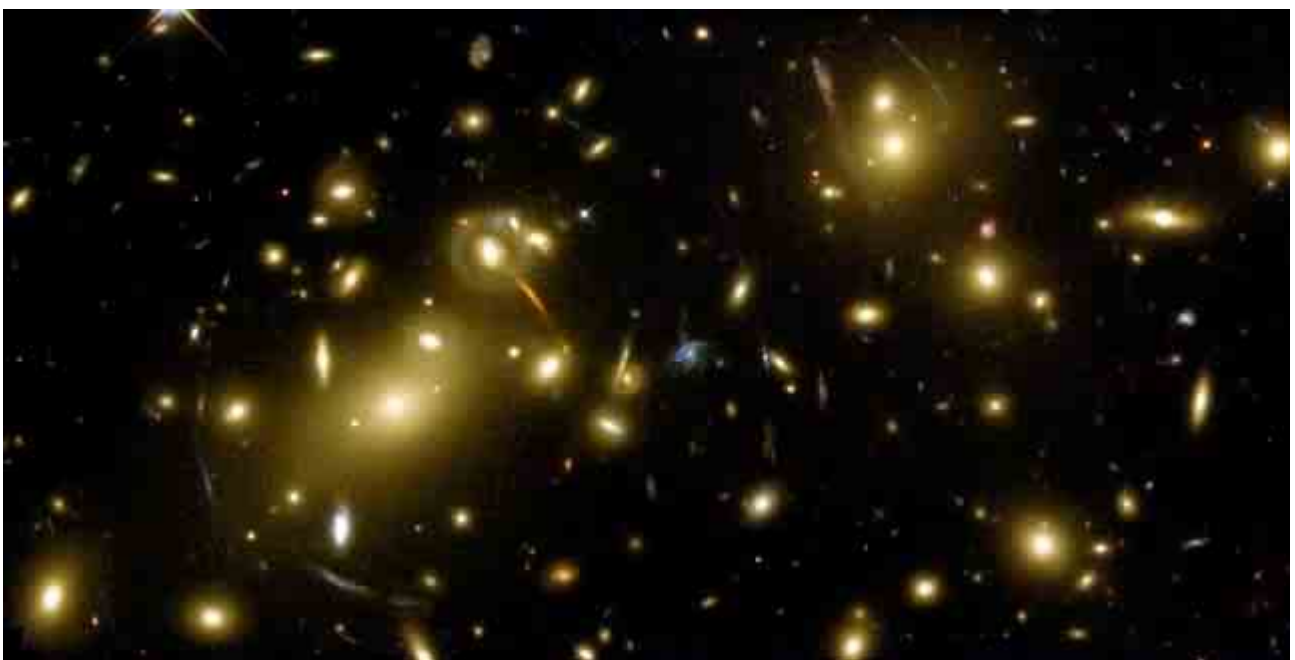
Galactische Cluster Abell 2218, gezien door Hubble Space Telescope. Bron: NASA. A. Fruchter and the ERO Team
